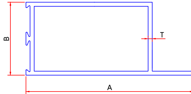
DOOR BOTTOM SINGLE LEG
